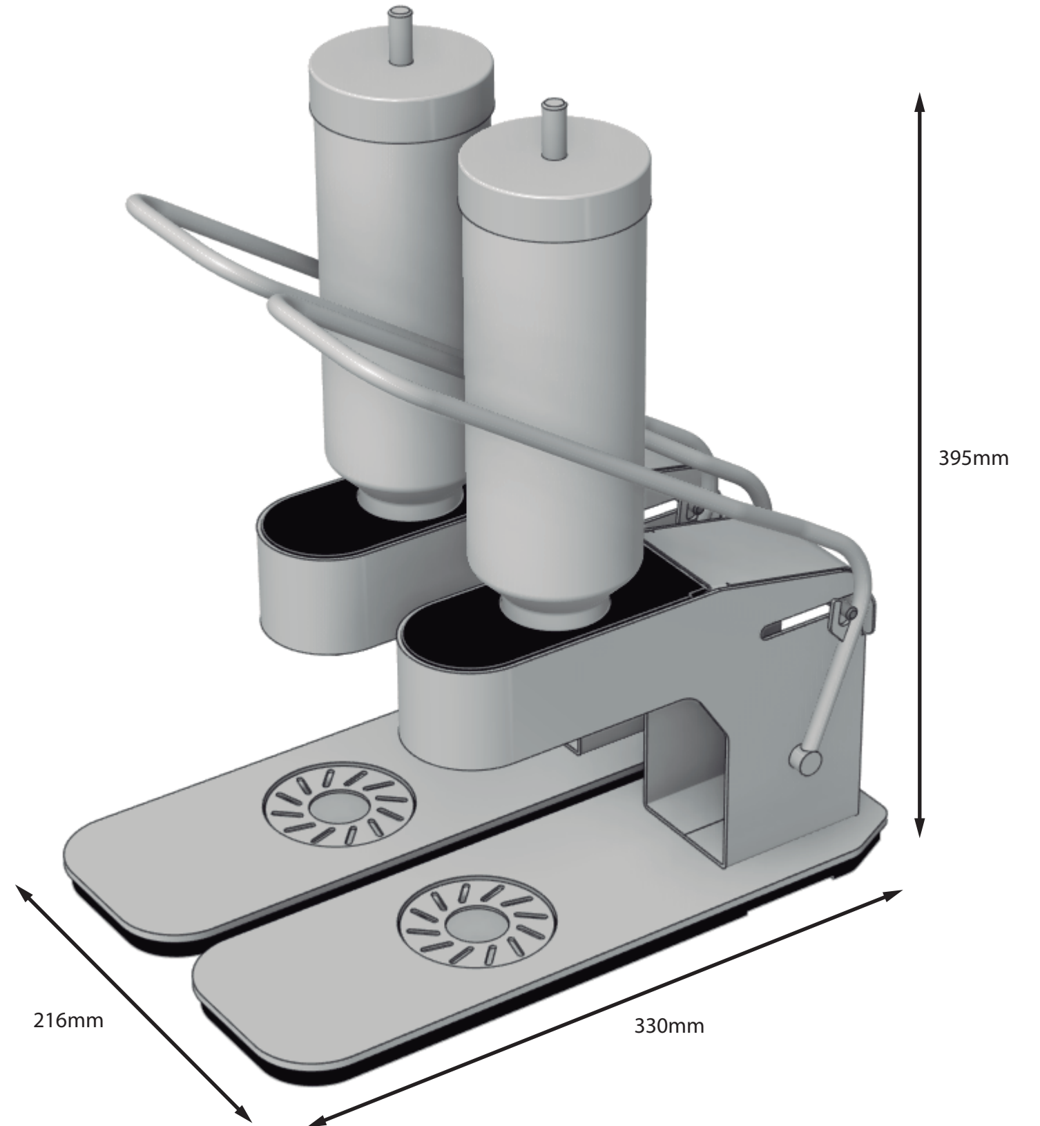
DISPENSADOR MERMELADA DOBLE: Medidas generales
